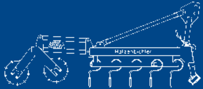
Nivelatorfeld, 5-balkig mit geraden Garezinken mit Wendescharen.
